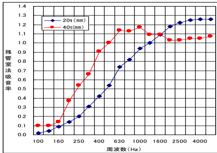
巻付け耐火被覆材の吸音率
